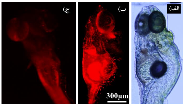
شکل ۶: تصاویر فلورئوسانس بدست آمده از رویان ماهی زبرا. الف) تصویر رویان ماهی زبرا توسط میکروسکوپ عبوری. توجه شود که با اینکه یک چشم ماهی در عقب قرار دارد هنوز مشاهده می‌شود ب) تصویر فلورئوسانس یک صفحه از این رویان. ج) تصویر سه بعدی بدست آمده از یک رویان دیگر با میکروسکوپ ساخته شده.
