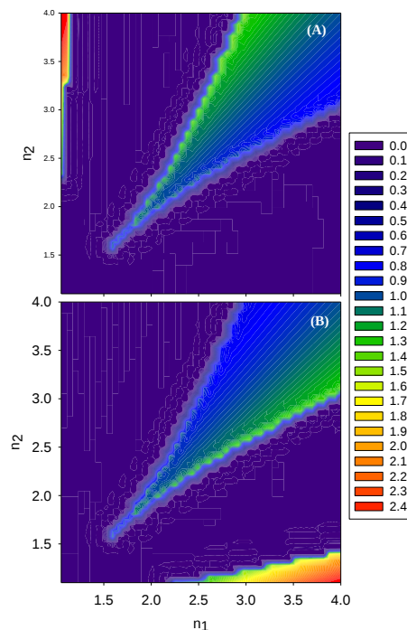
شکل ۲: نقشه خطای نسبی اندازه گیری در یک OPL محیط دو لایه برای بازه وسیعی از ضریب شکست. (A) لایه اول و (B) لایه دوم
