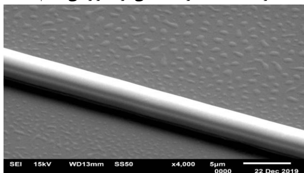
شکل (۲): تصویر SEM موجبر SU8 ساخته شده
