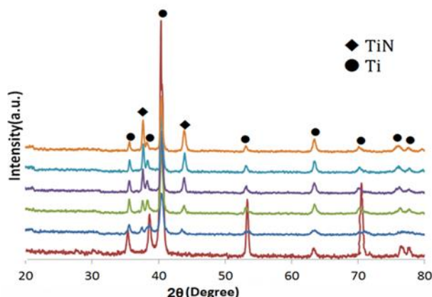
شکل ۳: الگوهای پراش اشعه ایکس فلز مرجع تیتانیوم S0(a) و نمونه‌های پرتودهی شده S1(b)، S2(c)، S3(d)، S4(e) و S5(f).
