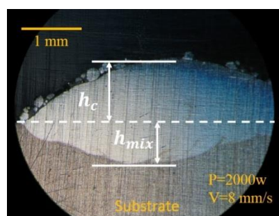
شکل ۳: تصویر سطح مقطع عرضی پوشش ایجاد شده با بزرگنمایی ۵.
