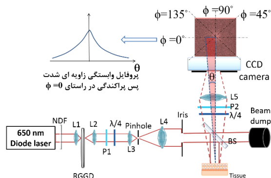
شکل ۴: آرایه اندازه گیری EBS. NDF: فیلتر چگالی خنثی، P: قطبشگر خطی، L: لنز، BE: پرتو گسترده، BS: مقسم پرتو.
