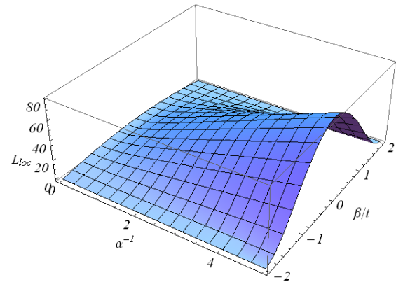
شکل ۲: طول جایگزیدی ( L_{loc} ) برحسب ثابت انتشار ( \beta ) و شعاع همبستگی ( \alpha^{-1} ) برای آرایه یک بعدی از موجبرها با ثابت های انتشار همبسته کوتاه برد نمایی.
