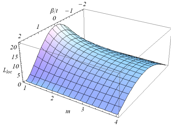
شکل ۳: طول جایگزیدی ( L_{loc} ) برحسب ثابت انتشار ( \beta ) و معکوس قدرت همبستگی ( m ) در آرایه یک بعدی از موجبرها با ثابت های انتشار همبسته بلند برد.
