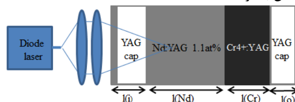
شکل (۱): شمایی از سیستم میکرولیزر سوئیچ Q انفعالی توان بالا با دمش دیودی
