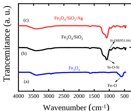
شکل ۲. طیف FTIR مربوط به نانوذرات \text{Fe}_3\text{O}_4 (منحنی آبی). \text{Fe}_3\text{O}_4/\text{SiO}_2 (منحنی سیاه) و \text{Fe}_3\text{O}_4/\text{SiO}_2/\text{Ag} (منحنی قرمز)
