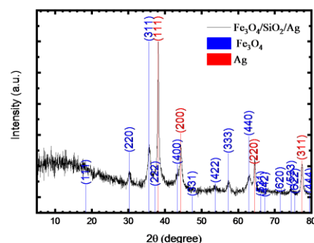
شکل ۱. طیف XRD نانوذرات مگنتیت/سیلیکا/نقره مربوط به نمونه S1.
