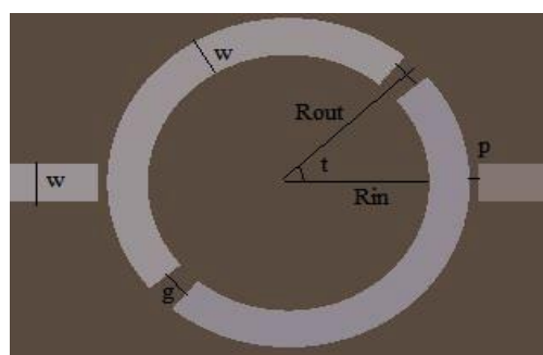
شکل ۱- ساختار فیلتر پلاسمونیکی پیشنهادی
