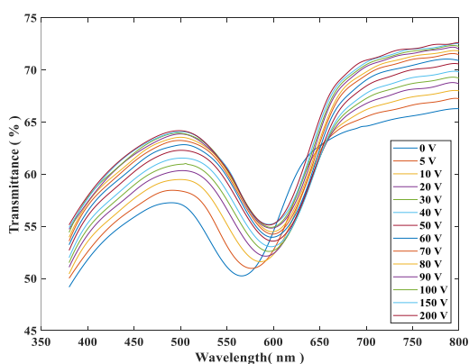
شکل (۳): جابجایی طیفی انعکاس انتخابی براگ برای نمونه ی بلورماید کستریک تثبیت شده در پلیمر در حضور میدان الکتریکی
