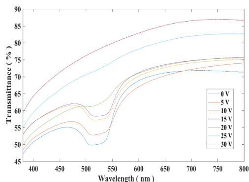
شکل (۱): جابجایی بازتاب براگ و تغییرات عبور نور برای نمونه ی بلورماید کستریک در حضور میدان الکتریکی خارجی
