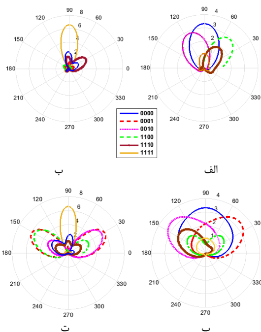
شکل ۴: نتایج شبیه‌سازی آنتن شکل (۱-ت)، الف و ب) نمودار الگوی تشعشعی در فرکانس تشدید 1THz، پ و ت) در فرکانس تشدید 1.3THz و به ترتیب در صفحات E و H
