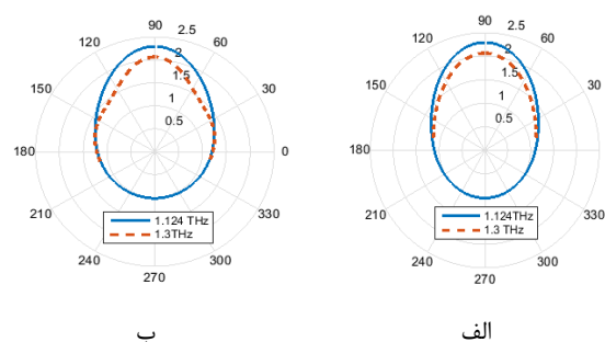
شکل ۲: (الف) الگوی تشعشعی در صفحه E و (ب) الگوی تشعشعی در صفحه H آنتن شکل ۱-الف در دو فرکانس کاری ۱/۱۲۴ و ۱/۳ تراهرتز
