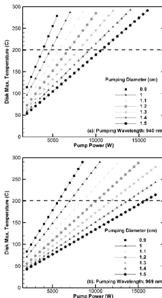
شکل ۳: دمای بیشینه دیسک بر حسب قطر لکه دمش، در توانهای دمش مختلف. برای طول موج دمش: (a) ۹۴۰ نانومتر و (b) ۹۶۹ نانومتر.
