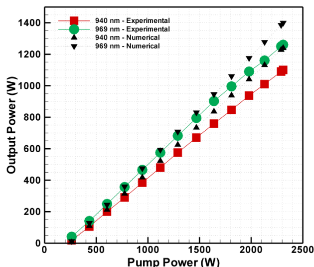
شکل ۵- منحنی توان خروجی لیزر بر حسب توان دمش.
