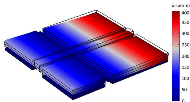
شکل ۳: چرخش کلید پیشنهادی در اثر تحریک الکترواستاتیک.
