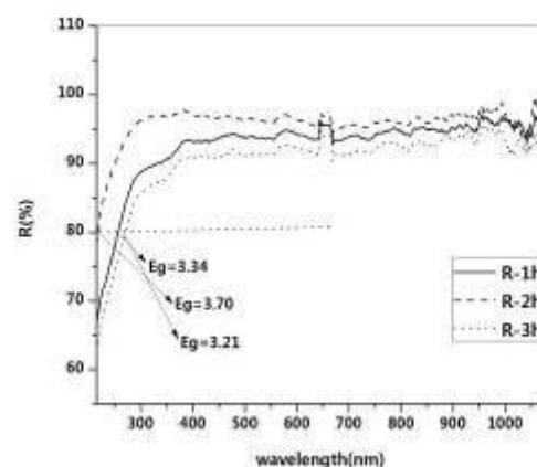
شکل ۳: طیف بازتابی
