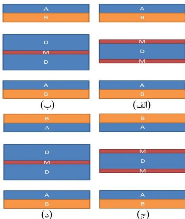
شکل ۱: تصویر شماتیک بلور فوتونی با نقص (الف) \{(AB)^p \text{ MDM } (AB)^q\} ، (ب) \{(AB)^p \text{ DMD } (AB)^q\} ، (ج) \{(BA)^p \text{ MDM } (AB)^q\} و (د) \{(BA)^p \text{ MDM } (AB)^q\}
