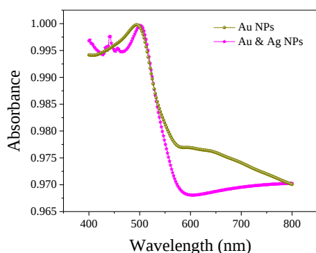
شکل ۳: طیف جذب برای نانوذرات طلا و برای دوپار نانوذرات طلا و نقره.
