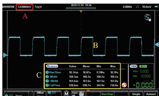
شکل ۳: نمایی از خروجی اسیلوسکوپ دیجیتال متصل به حسگر فوق سریع (A) : (Volt/Div = 10mV, Time/Div = 200μs) فرکانس قطار پالس لیزر، (B) نمای پالس مدوله شده روی لیزر دیودی، (C) اطلاعات مربوط به پالس همچون پهنا و زمان خیز/افت.
