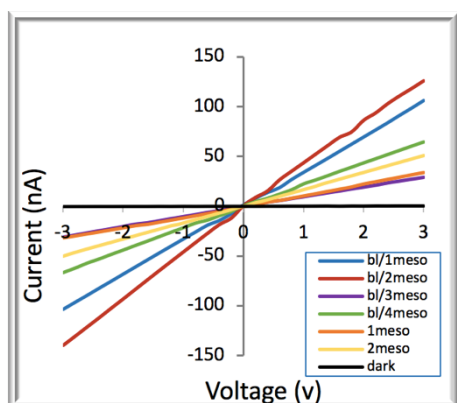
شکل ۲: نمودار جریان-ولتاژ آشکارساز نوری پروسکایت با ساختارهای مختلف در تاریکی و تحت تابش LED آبی ۴ ولت.
