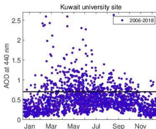
شکل ۲: عمق‌اپتیکی میانگین روزانه هواویزها در طول موج 440 nm از سال ۲۰۰۶-۲۰۱۸
