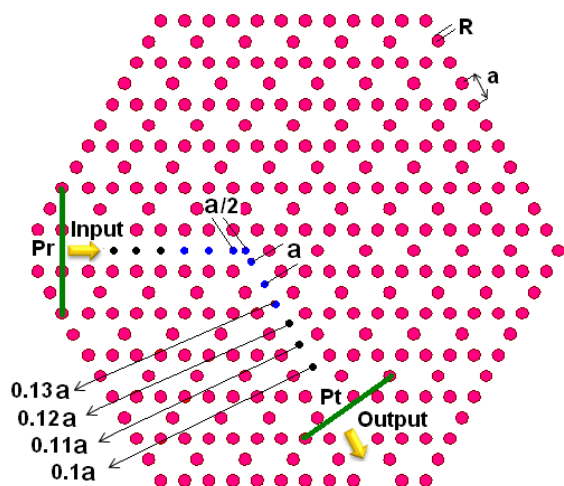
شکل ۲: ساختار نواری پیشنهادی برای خم موجبری ۶۰ درجه در شبکه ی بلور فوتونی کاگومه. این ساختار شامل ۴ میله ی اضافی در داخل موجبر می باشد که شعاع آن ها به صورت تدریجی و برابر با ۰.۱۳a، ۰.۱۲a، ۰.۱۱a، ۰.۱a تغییر می یابد.
