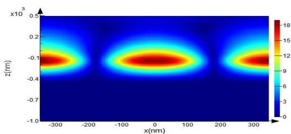
شکل ۲. توزیع میدان الکتریکی در فرکانس تشدید ساختار.
