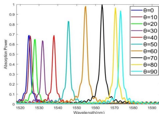
شکل ۳. نمودار طیف جذب جاذب نوری تنظیم‌پذیر بر حسب \theta های متناسب با ولتاژ اعمالی به کریستال مایع.
