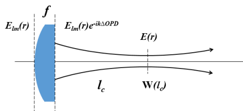
شکل ۴. اصول محاسبه قطر لکه کانونی در حضور ابیراهی کروی
