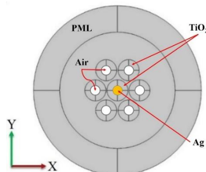
شکل ۳: هندسه مربوط به شبیه‌سازی به کمک بسته نرم‌افزاری کامسول شامل نانولوله‌های \text{TiO}_2 ، نانولوله مرکزی حاوی نقره می‌باشد. یک لایه‌ی جاذب کامل (PML) در سطح بیرونی جهت حذف پراکندگی غیر واقعی از لبه‌های خارجی در نظر گرفته شده‌است.
