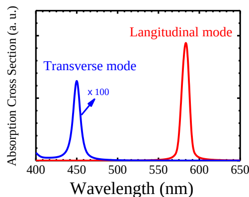
شکل ۵: طیف سطح مقطع جذب، در دو مد طولی (منحنی قرمز) و عرضی (منحنی سیاه)، ساختار هسته-پوسته‌ی استوانه‌ای \text{Ag@TiO}_2 برای مقایسه‌ی بهتر طیف مربوط به مد عرضی ۱۰۰ برابر شده است.
