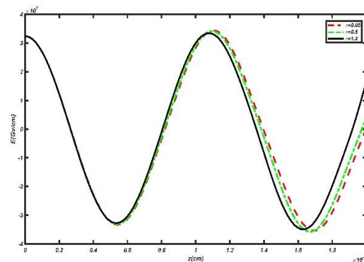
شکل ۲ ( میدان الکتریکی در حالت اتلاقی برای فرکانس های برخورد مختلف:
