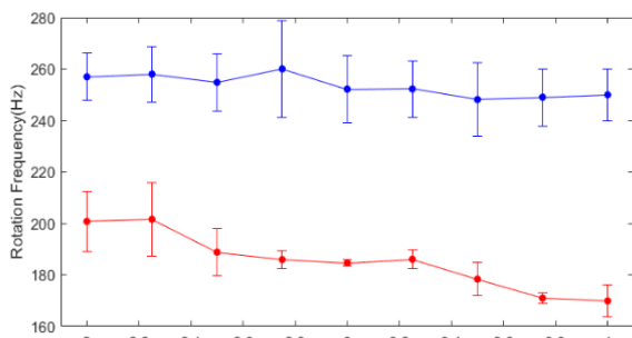
شکل ۴: نمودار تغییرات سرعت چرخش ذره اول با دور شدن ذره دوم بر حسب فاصله بین دو ذره را نشان می‌دهد. داده‌های آبی و قرمز به ترتیب مربوط به قطبش موازی و عمود بر خط واصل دو ذره است.
