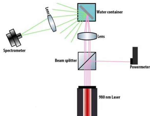
شکل ۲: نمای کلی از چیدمان اپتیکی اندازه گیری فلورسانس نانوتابشگرهای تبدیل افزایشی که شامل لیزر ۹۸۰ نانومتر، جداکننده باریکه، توان سنج، عدسی‌ها، محفظه آب و طیف سنج است. درجه سانتی‌گراد به مدت یک ساعت قرار گرفت تا فرآیند
