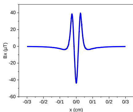
شکل ۱-۳ الف: توزیع میدان مغناطیسی در راستای x ، 0.1\text{ cm} زیر پیچه‌ها
