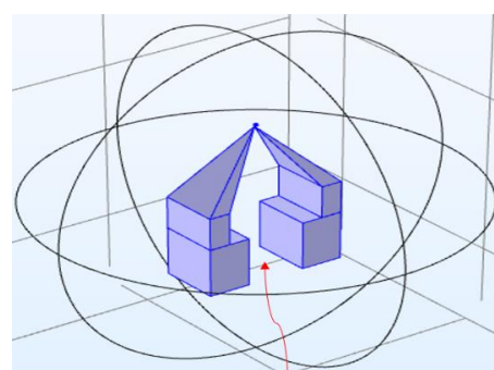
جایگاه مغناطومتر اتمی ( 1/4\text{ cm} )
