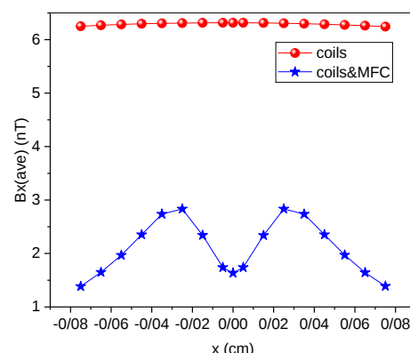
نمودار ۶-۱: مقایسه اثر متمرکز کننده شار مغناطیسی بر تفکیک پذیری
