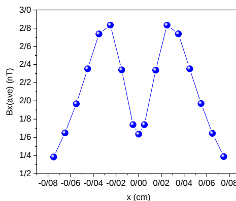
نمودار ۵-۱: میدان مغناطیسی محاسبه شده در راستای x با استفاده از متمرکز کننده شار مغناطیسی
