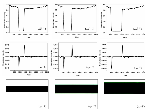
شکل ۵. سیگنال جسم (الف)، سیگنال مشتق (ب) و تصویر آشکارساز ماتریسی (پ) مربوط به جسمی به قطر 3/992 میلیمتر (۱) جسمی به قطر 5/994 میلیمتر (۲) و مربوط به جسمی به قطر 7/986 میلیمتر (۳).
