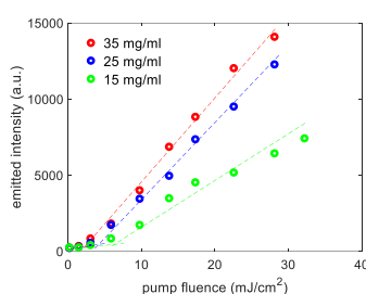
شکل ۶: منحنی‌های شدت تابشی بر حسب چگالی انرژی دمش.
