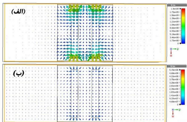
شکل ۳. شبیه‌سازی بردار میدان الکتریکی در دو فرکانس متفاوت؛ (الف) در فرکانس تشدید 235\text{ THz} و (ب) در فرکانس غیرتشدید 224\text{ THz} .
