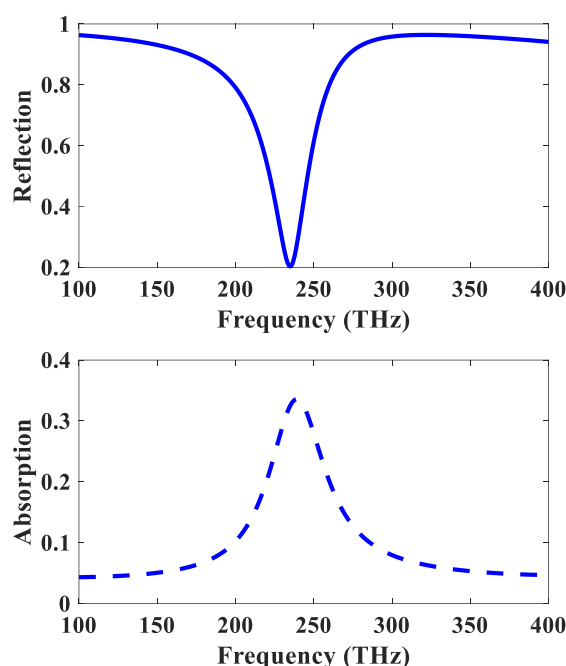
شکل ۲. نمودار طیف بازتاب و طیف جذب از ساختار. در این حالت در فرکانس 235\text{ THz} ، گافی در طیف بازتاب و قله‌ای در طیف جذب مشاهده می‌شود که نشان‌دهنده برهم‌کنش تشدیدی ساختار با موج الکترومغناطیسی فرودی در این فرکانس است.
