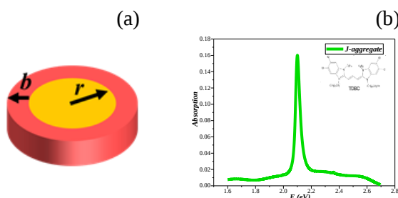
شکل ۱: (a) شمای ساختار هیبرید، (b) طیف جذب لایه‌ی مولکول تجمع یافته TDBC [۱۳]
