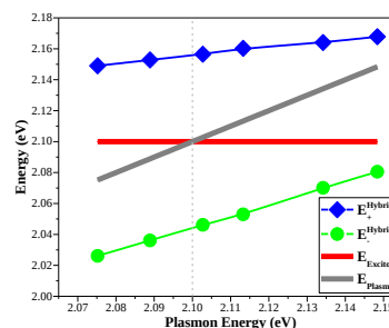
شکل ۵: تغییرات انرژی مدهای هیبریدی (منحنی آبی و سبز رنگ) به ازای تغییر انرژی پلاسmoni. منحنی قرمز و طوسی نشانگر انرژی مد های غیر هیبریدی اکسایتونی و پلاسmoni می باشد.
