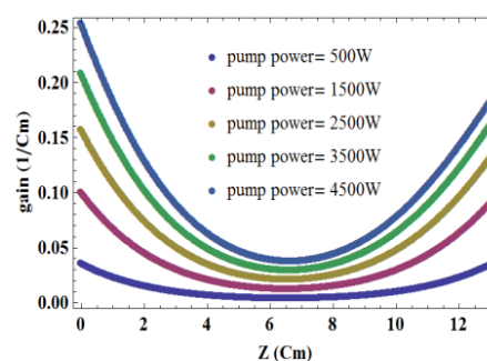
شکل ۳: توزیع ضریب بهره در طول کریستال در تقویت کننده تیغه ای زیگزاگ به ازای توان‌های مختلف در هر سر تیغه
