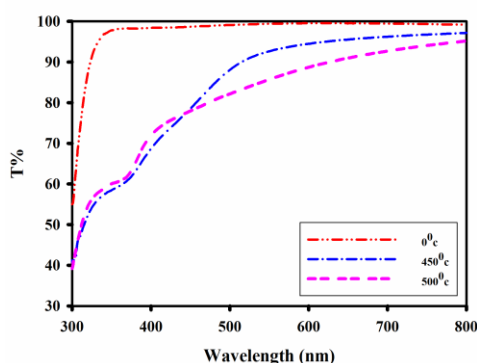
شکل ۳: طیف تراگیسل نمونه های بدون بازپخت و بازپخت شده در دماهای ۴۵۰، ۵۰۰ درجه سانتیگراد.
