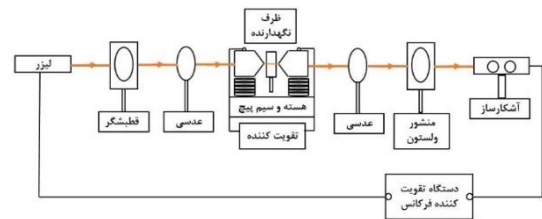
شکل ۴: طرحواره‌ی از چیدمان فارادی.
