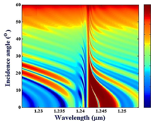
شکل ۴. وابستگی بازتابندگی بلور تک نقص به زاویه تابش. نمودار رنگی بازتابندگی بر حسب طول موج برای زاویه های مختلف را نمایش می دهد. دمای بلور 10\text{ K} در نظر گرفته شده است.
