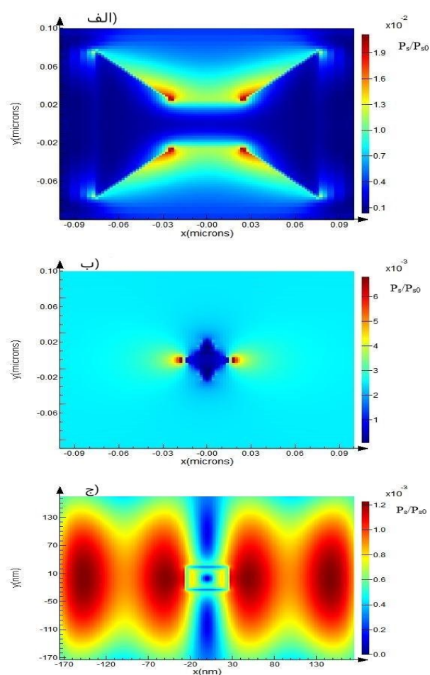
شکل ۴: توان‌های خروجی در ساختار الف) مرجع (ب) ستاره‌ای چهارپر ج) هشت‌وجهی ساده
