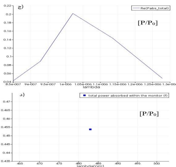
شکل ۵: الف) توان جذب شده در واحد حجم مرجع (ب) توان جذب شده در واحد حجم ساختار هشت وجهی با لنز پلاسمونیک که افزایش ۱۰ برابری را نشان می‌دهد ج) توان جذبی کل بهنجار مرجع د) توان جذبی کل بهنجار ساختار هشت وجهی با لنز پلاسمونیک که در تک طول موج بررسی شد.
