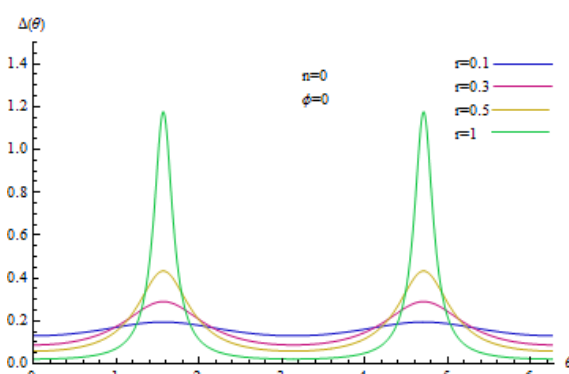
شکل ۲: شاخص \Delta(\theta) برای حالت فشرده فوتونی، n = 0 ، و زاویه فشردگی \phi = 0 ثابت، برای پارامتر فشردگی متفاوت r = 0.1, 0.3, 0.5, 1 .
