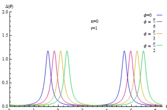
شکل ۳: شاخص \Delta(\theta) برای حالت فشرده فوتونی، n = 0 ، و پارامتر فشردگی r = 1 ثابت، برای زاویه فشردگی متفاوت \phi = 0, \pi/2, \pi/3, \pi/6 .
