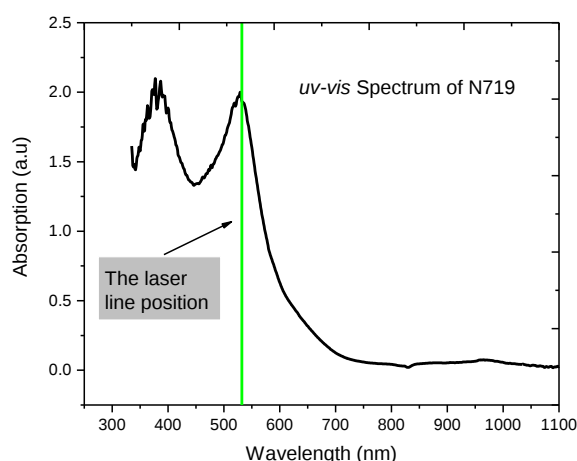
شکل ۲: طیف UV – VIS نمونه N719 حل شده در اسیتونیتریل
