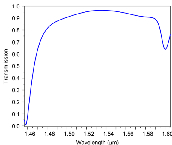
شکل ۳: بهره‌ی طیف عبوری خم موجبر نشان داده شده در شکل ۲.
