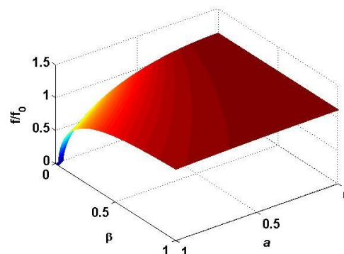
شکل ۶: تغییرات شعاع لکه \frac{f}{f_0} برای باریکه لیزری قطبیده دایروی چیگرد بر حسب a و \beta برای \frac{z}{z_R} = 0.5
