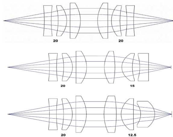
شکل ۴: سامانه های نوری موازی کننده و کانونی کننده
