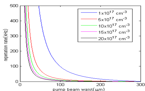
شکل ۲: تغییرات انرژی تیپ، پهنای تیپ و نرخ تکرار بر حسب شعاع پرتو دمش به ازای غلظت های مختلف آلایش جاذب اشباع پذیر
