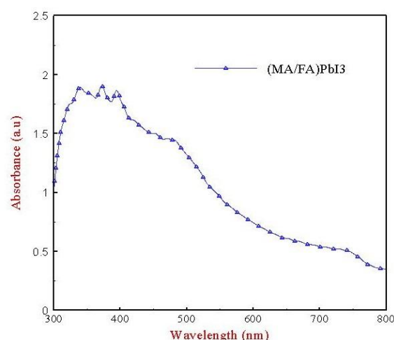
شکل ۵: طیف جذب (UV-Visible) از (MA_{1-x}FA_xPbI_3)
