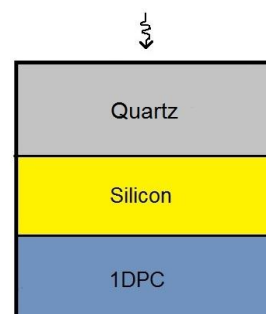
شکل ۱: نمایی از ساختار طراحی شده برای افزایش جذب نور در لایه‌ی سیلیکون.
