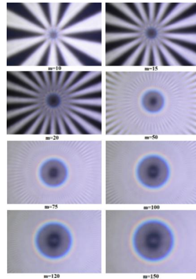
شکل ۲: طرح‌های پراش برای توری‌های شعاعی رانگی با تعداد پره‌های مختلف. توری‌ها در فاصله Z=80 سانتی از دوربین قرار گرفته‌اند. با بالا رفتن تعداد پره‌ها، شعاع حلقه‌های رنگی طبق رابطه ۴ افزایش پیدا می‌کند.
