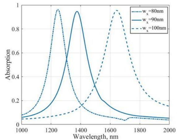
شکل ۵: (الف) نمودار طیفی جذب به ازای مقادیر مختلف p_x
