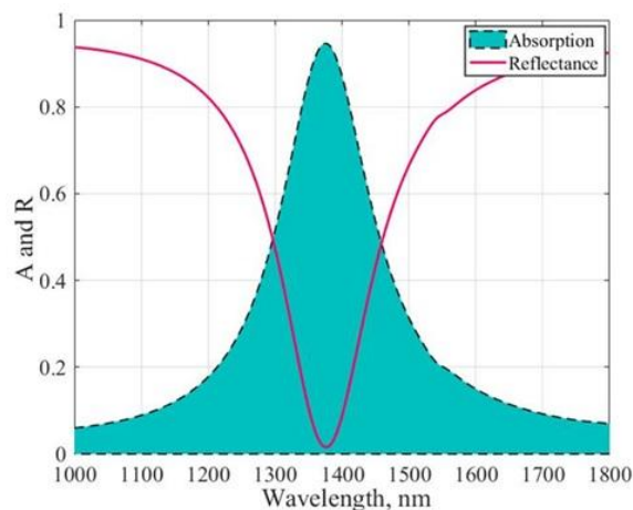
شکل ۳: نمودار طیفی جذب و بازتاب فرامواد فلز-دی‌الکتریک-فلز
