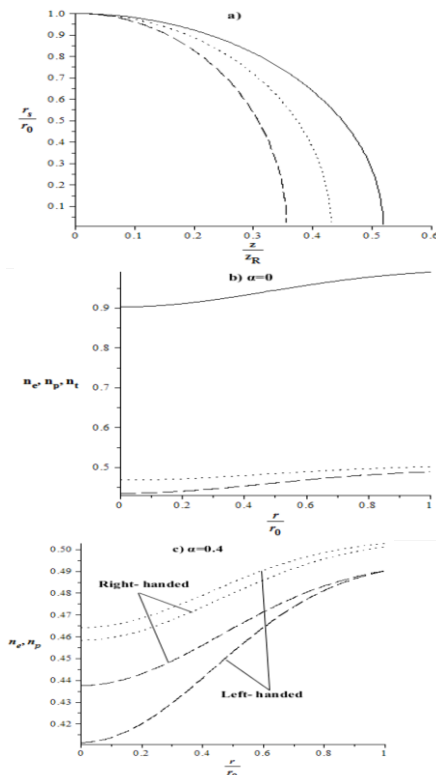
شکل (۴) (a) تغییرات r_s/r_0 بر حسب z/z_R (b) تغییرات چگالی نسبت به r/r_0 در حالت \alpha=0 (c) تغییرات چگالی الکترون و پوزیترون نسبت به r/r_0 در حالت \alpha=0.4
