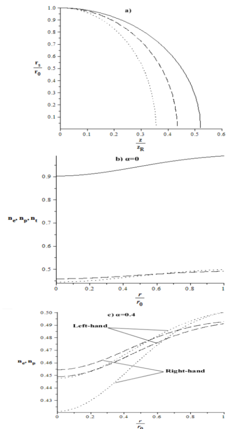
شکل (۴) (a) تغییرات r_s/r_0 بر حسب z/z_R (b) تغییرات چگالی نسبت به r/r_0 در حالت \alpha=0 (c) تغییرات چگالی الکترون و پوزیترون نسبت به r/r_0 در حالت \alpha=0.4
