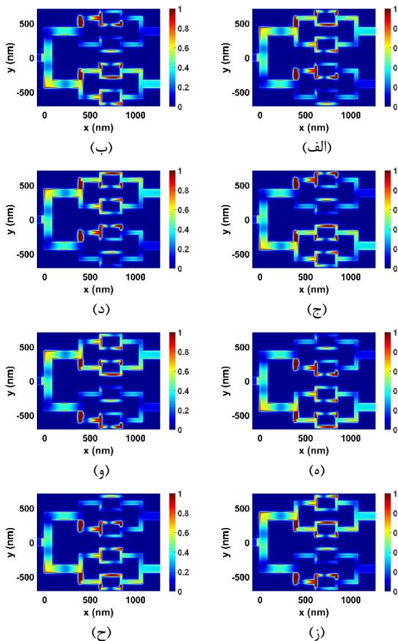
شکل ۲: نمایه‌ی میدان الکتریکی به ازای حالت‌های مختلف ورودی (الف) A=B=C=0 (ب) A=B=0, C=1 (ج) A=C=0, B=1 (د) A=0, B=C=1 (ه) A=1, B=C=0 (و) A=C=1, B=0 (ز) A=B=1, C=0 و (ح) A=B=C=1
