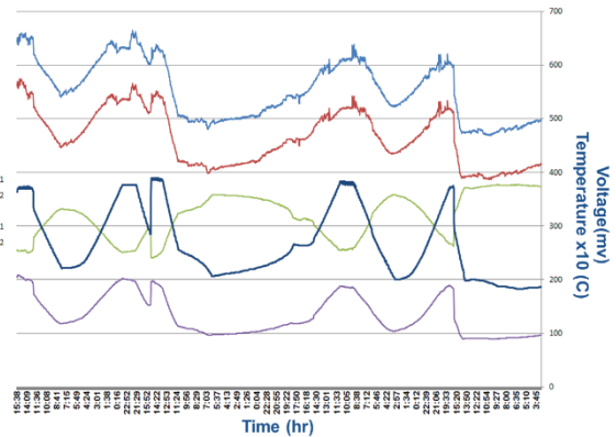
شکل ۲: تغییرات مقادیر ac_1 , ac_2 , dc_1 , dc_2 نسبت به تغییرات دما در ولتاژ ثابت
