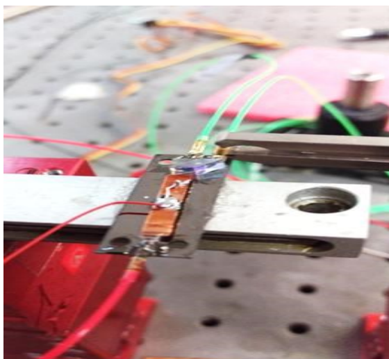
شکل ۱: ساختار حسگر نوری ولتاژ دو خروجی برپایه نگه‌دارنده سیلیکون
